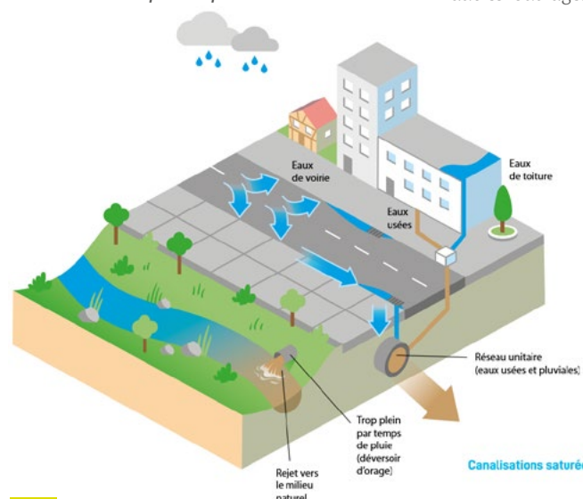
Le réseau unitaire, modèle le plus répandu en Alsace
